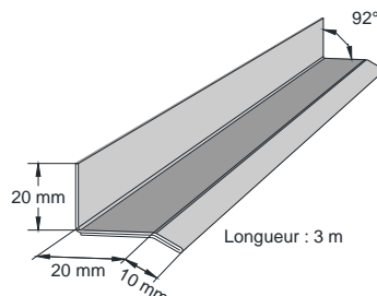
Larmier de 20
