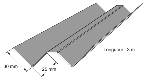
Coin intérieur continu
